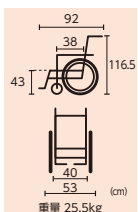
MH-CR2のサイズ となります ティルト角度 0 ~ 30° リクライニング角度 90 ~ 125°
