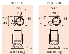
NEXT-11B (自操式)
