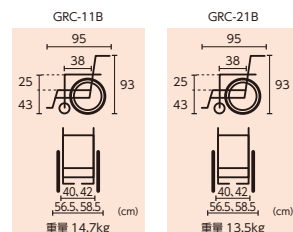
GRC-11B (自操式)
