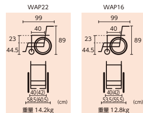
WAP22 (自操式)
