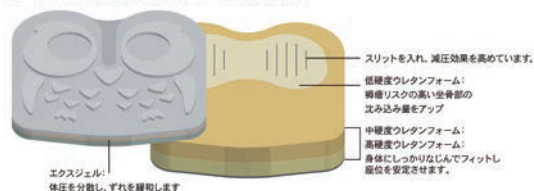
■ エクスジェルとウレタンフォームの積層構造
